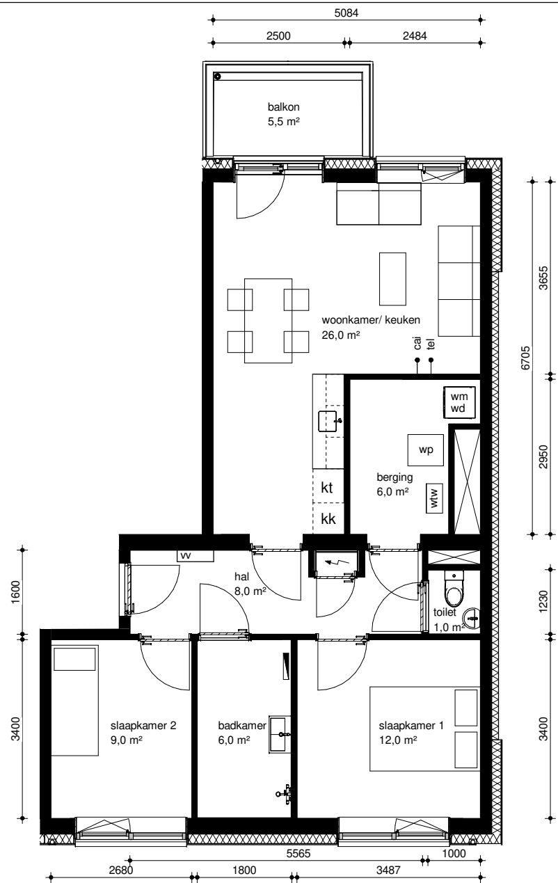
plattegrond type G 2
